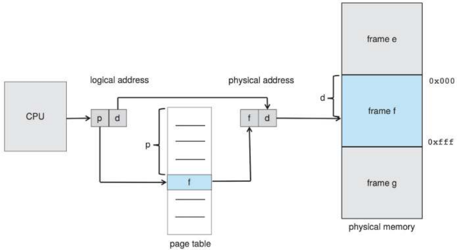
Figure 9.8 Paging hardware.
